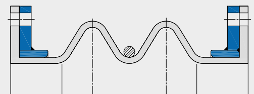
Beispiel - 2-wellig, Ausführung A - unverspannt
