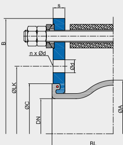
Ausführung S zugverspannt/schubbegrenzt mit Kugelscheiben/Kegelpfannen
