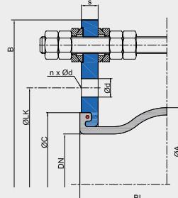
Ausführung M zugverspannt/schubbegrenzt mit Kugelscheiben/Kegelpfannen
