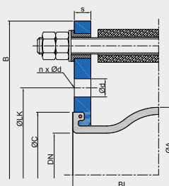
Ausführung S zugverspannt/schubbegrenzt mit Kugelscheiben/Kegelpfannen
